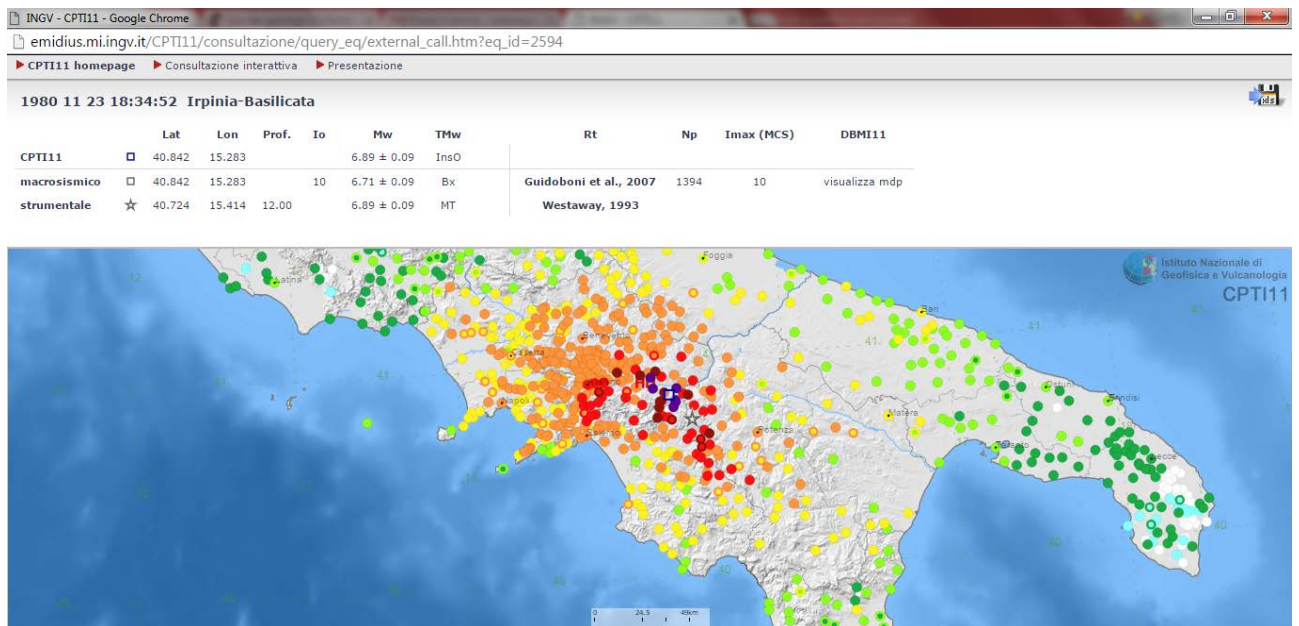
Catalogo Parametrico dei Terremoti Italiano CPTI11
