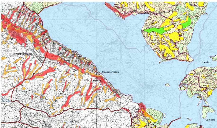
Screenshot Aree a pericolosità da frana – Comune di Magliano Vetere
